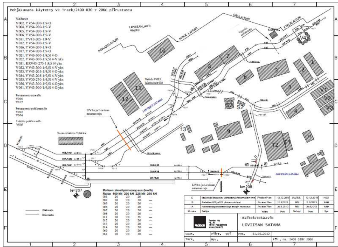
Liite 2: Raiteistokaavio
