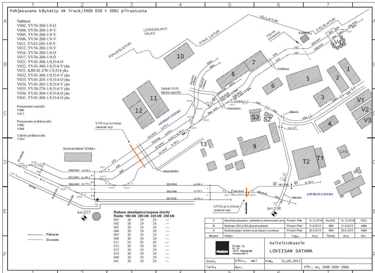
Liite 2: Raiteistokaavio
